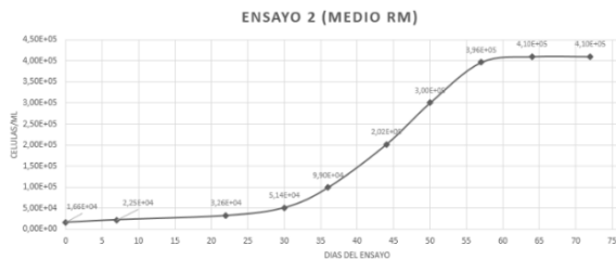
Figura 5. Curva de crecimiento celular en medio de cultivo RM
