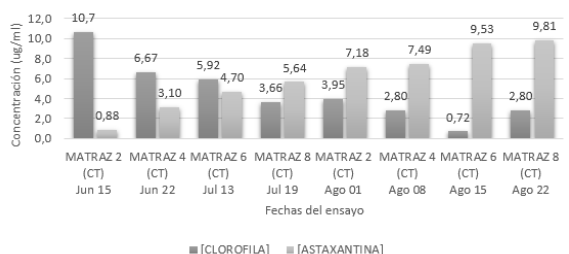
Figura 4. Cuantificación de clorofila y astaxantina del ensayo 1 en medio de cultivo BBM con tratamiento (ug/ml)
