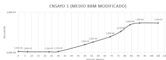
Figura 2. Curva de crecimiento celular en medio de cultivo BBM modificado (menor % nitrógeno)
