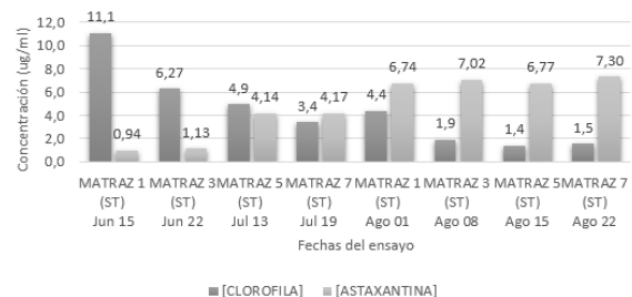
Figura 3. Cuantificación de clorofila y astaxantina del ensayo 1 en medio de cultivo BBM sin tratamiento (ug/ml)
