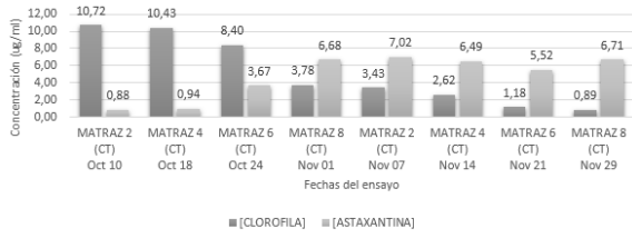
Figura 7. Cuantificación de clorofila y astaxantina del ensayo 2 en medio de cultivo RM con tratamiento (ug/ml)
