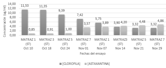
Figura 7. Cuantificación de clorofila y astaxantina del ensayo 2 en medio de cultivo RM con tratamiento (ug/ml)
